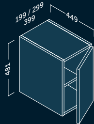
MÓDULO PUERTA REVERSIBLE
