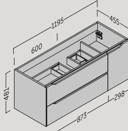
CENIT 120 (47.2") SENO CENTRADO
