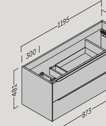
CENIT 120 (47.2") SENO DESPLAZADO
