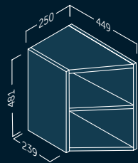
MÓDULO CHAFLÁN REVERSIBLE | FONDO 45 A 24
