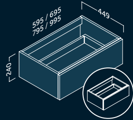
MÓDULO 1 CAJÓN SIN SALVASIFÓN NI ORGANIZADOR
