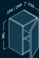
MÓDULO PUERTA REVERSIBLE | FONDO 24
