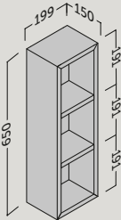
ESTANTE X3 VERTICAL
