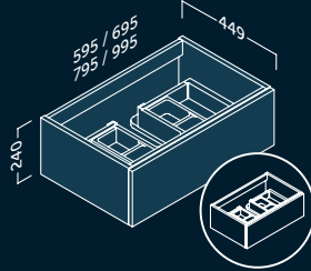
MÓDULO 1 CAJÓN CON SALVASIFÓN Y ORGANIZADOR
